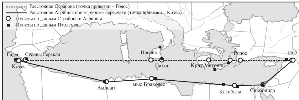
Рис. 3. Сведения Страбона и Агриппы в сравнении с картой Птолемея
