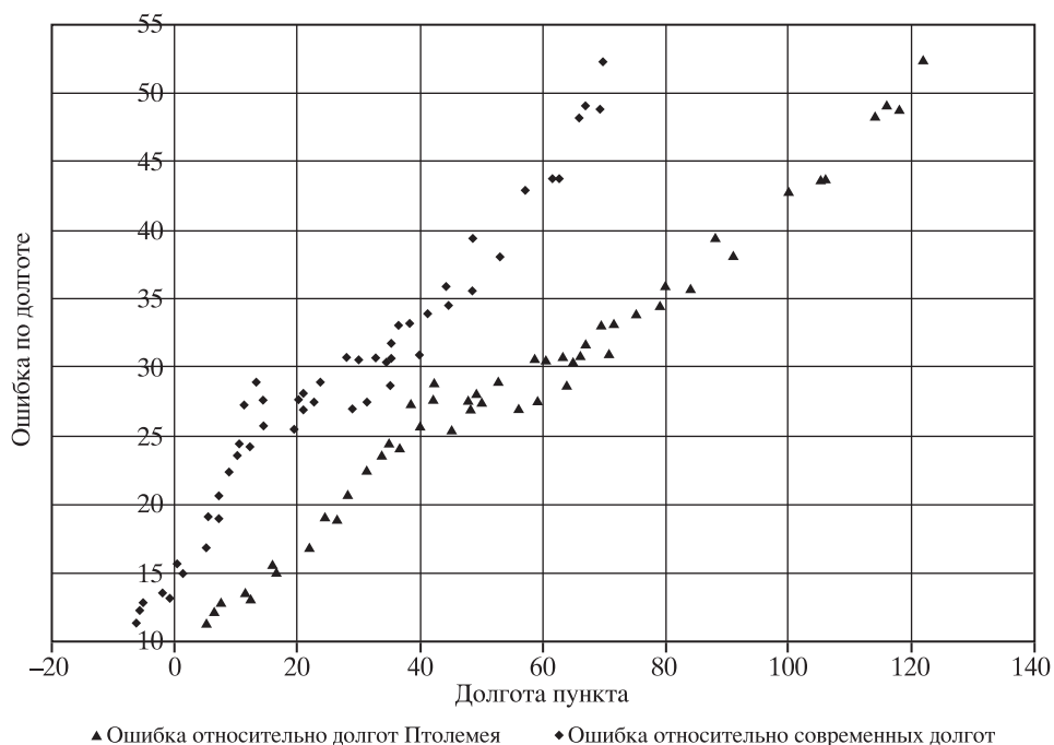
Рис. 4. Ошибка по долготе на карте Птолемея
